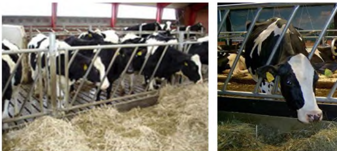
Рисунок 5 - Диагональная кормовая решетка при беспривязном содержании коров (© ЭкоАгро, 2013)
