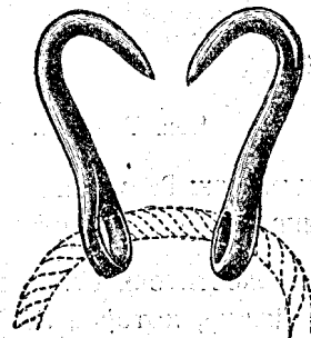
Крючки Гармса.
