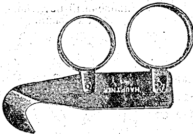
Нож Тапкена.
