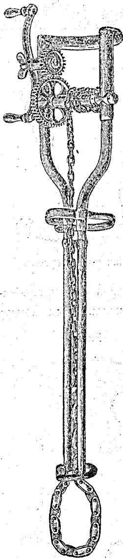
Эмбриотом Пфланца.
