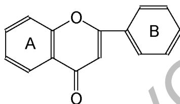
Флаванон
