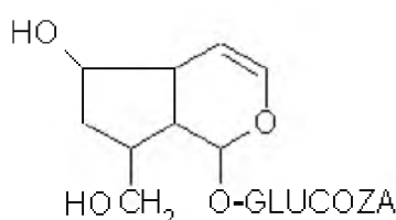
Аукубин
