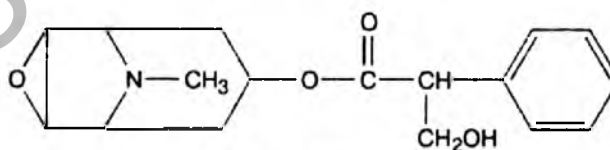
Скополамин
