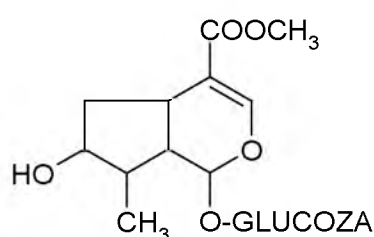
Логанин
