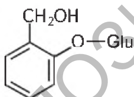
Салицин
