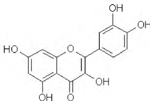
Кверцетин
