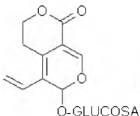
Генциопикрин
