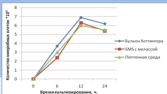
Рисунок 3. – Рост Bacillus megaterium на различных типах питательных сред
