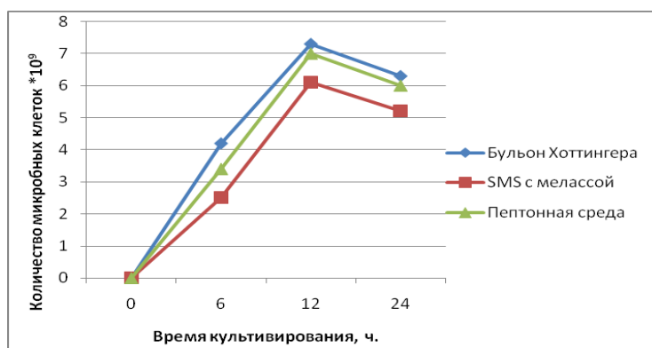
Рисунок 1. – Рост Bacillus subtilis на различных типах питательных сред
