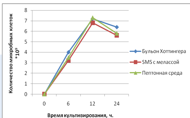
Рисунок 2. – Рост Bacillus licheniformis на различных типах питательных сред
